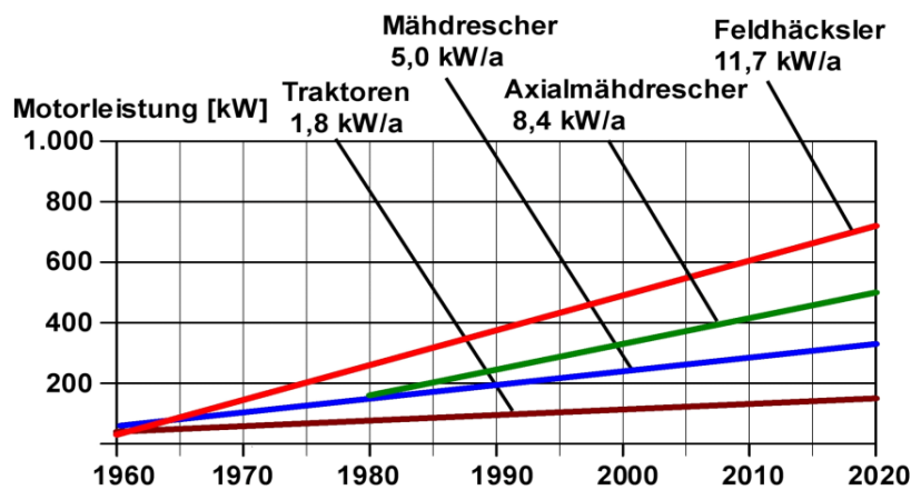
Bild 6: Steigerung der Motorleistung in kW/a für ausgewählte landtechnische Arbeitsmittel des mobilen Bereiches mit den durchschnittlichen jährlichen Steigerungsraten nach [5], die auch als „Wachstumsgesetz der Landtechnik“ bezeichnet wird.
