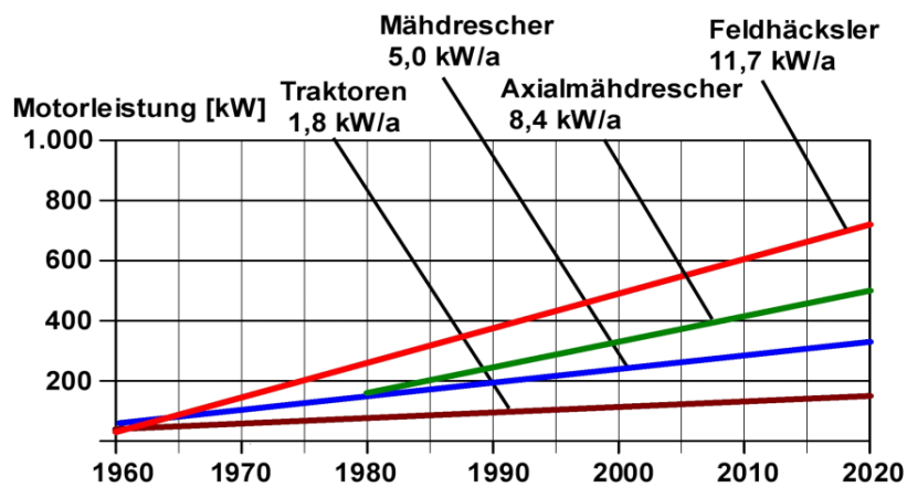
Bild 6: Steigerung der Motorleistung in kW/a für ausgewählter landtechnischer Arbeitsmittel des mobilen Bereiches mit den durchschnittlichen jährlichen Steigerungsraten nach [5], die auch als „Wachstumsgesetz der Landtechnik“ bezeichnet wird.
